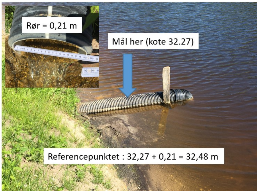
Figur 8.26 Opmåling af en dækket udløbskote
