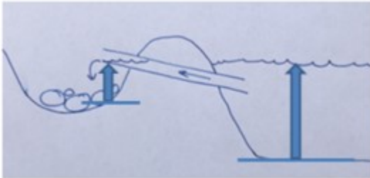
Figur 8.25 Eksempel på udløbsrør. Udløbskoten er i toppen af den venstre pil.
