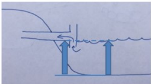
Figur 8.22 Eksempel på udløbsrør. Udløbskoten er i toppen af den venstre pil.
