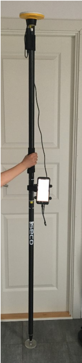
Figur 7.2 Trimble opmålingssæt. Præcisionen er 2-3 cm horisontal og 4 cm vertikal.
