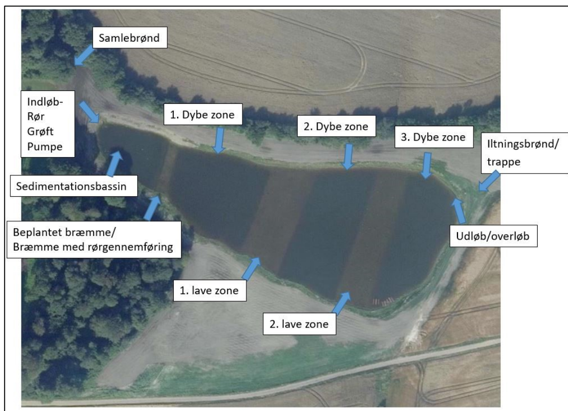
Figur 5.1 Oversigt over de forskellige elementer i et minivådområde
