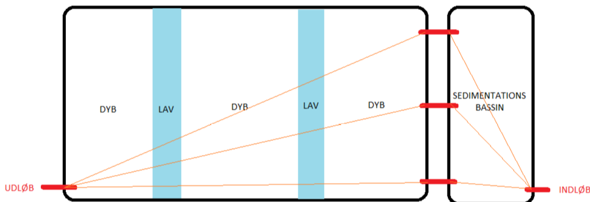
Figur 4.1 Eksempel på minivådområde med flere rør mellem sedimentationsbassin og minivådområdet.
