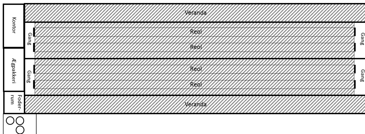
Figur 3.3.2. Eksempel på slagtekyllingestald, hvor kyllingerne opstaldes i det skraverede område, der er defineret som nettoproduktionsareal. Tilstødende faciliteter såsom service- og teknikrum, befæstede arealer mv. er ikke omfattet af nettoproduktionsarealet.
