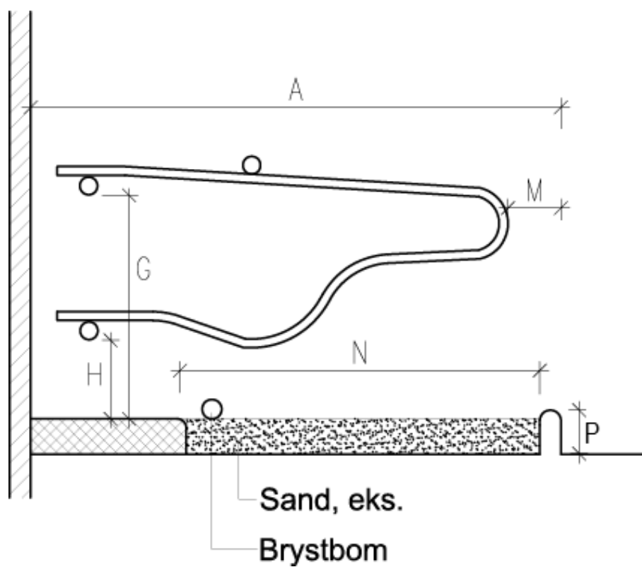
Figur 4 Anbefalede mål på sengebåse til kalve og ungkvæg i stalde bygget efter 1. juli 2010
