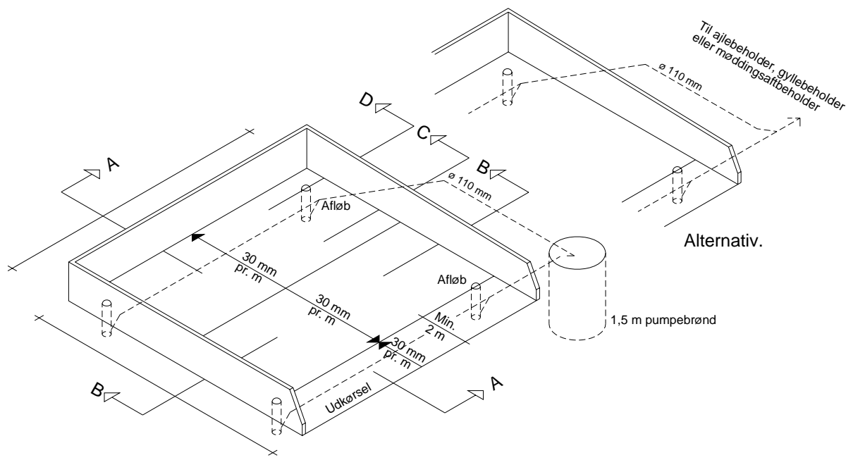
b) Figur 1.9 Eksempel på korrekt konstruktion af møddingsplads med afgrænsningsmur og fald mod afløb. Kilde: Landbrugets Byggeblade, Arkiv nr. 103.06-05
