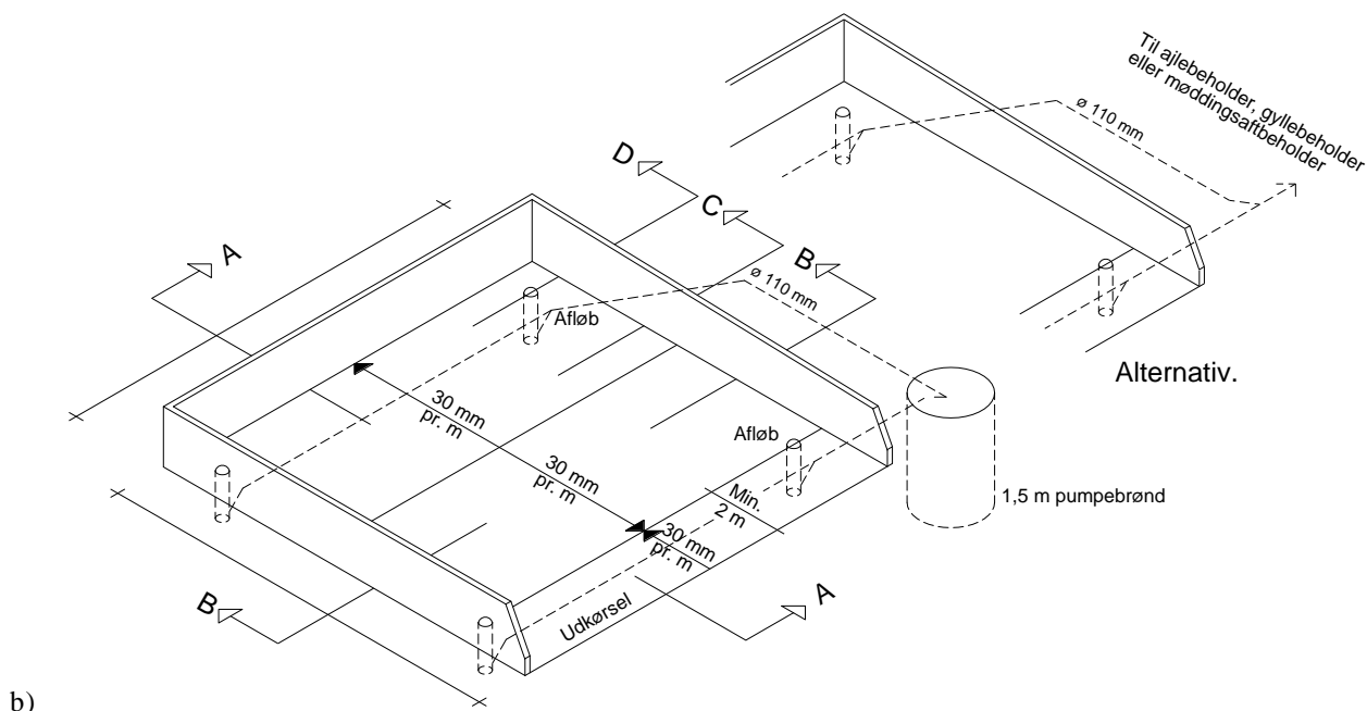
Figur 1.9 Eksempel på korrekt konstruktion af møddingsplads med afgrænsningsmur og fald mod afløb. Kilde: Landbrugets Byggeblade, Arkiv nr. 103.06-05
